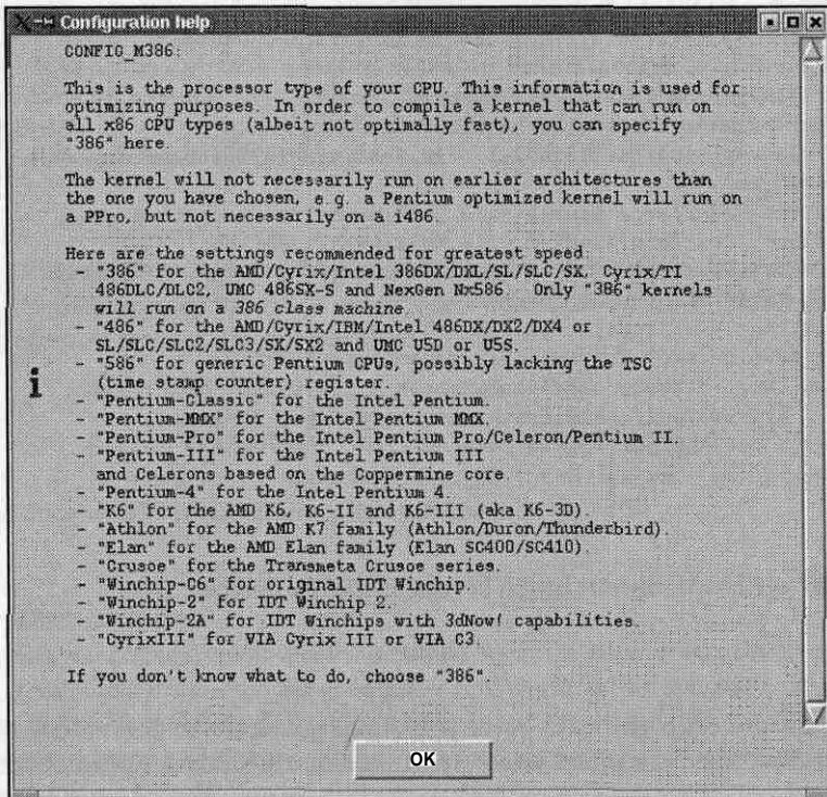
Figuur 1.6 Een van de help-vensters van het submenu 'processor'.
